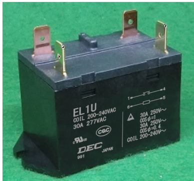
EL1U (タブ端子型)
